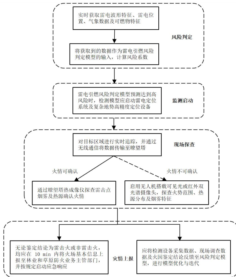
图 2 系统工作流程图
